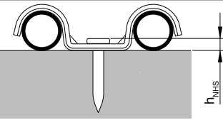
Fijación a acero, Fijación a hormigón
