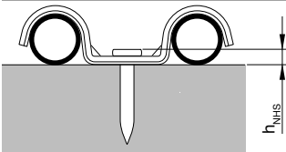
Fixation au béton, Fixation dans l'acier
