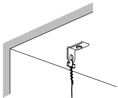
Elektrische und mechanische Befestigung an der Decke
