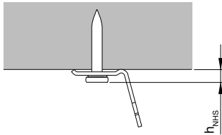
Fixation au béton, Fixation dans l'acier
